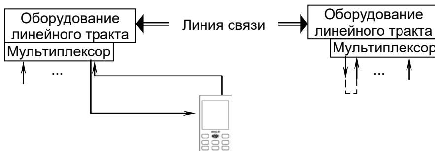
Рис. В1.2. Схема тестирования канала N×64 Кбит/с с использованием шлейфа
